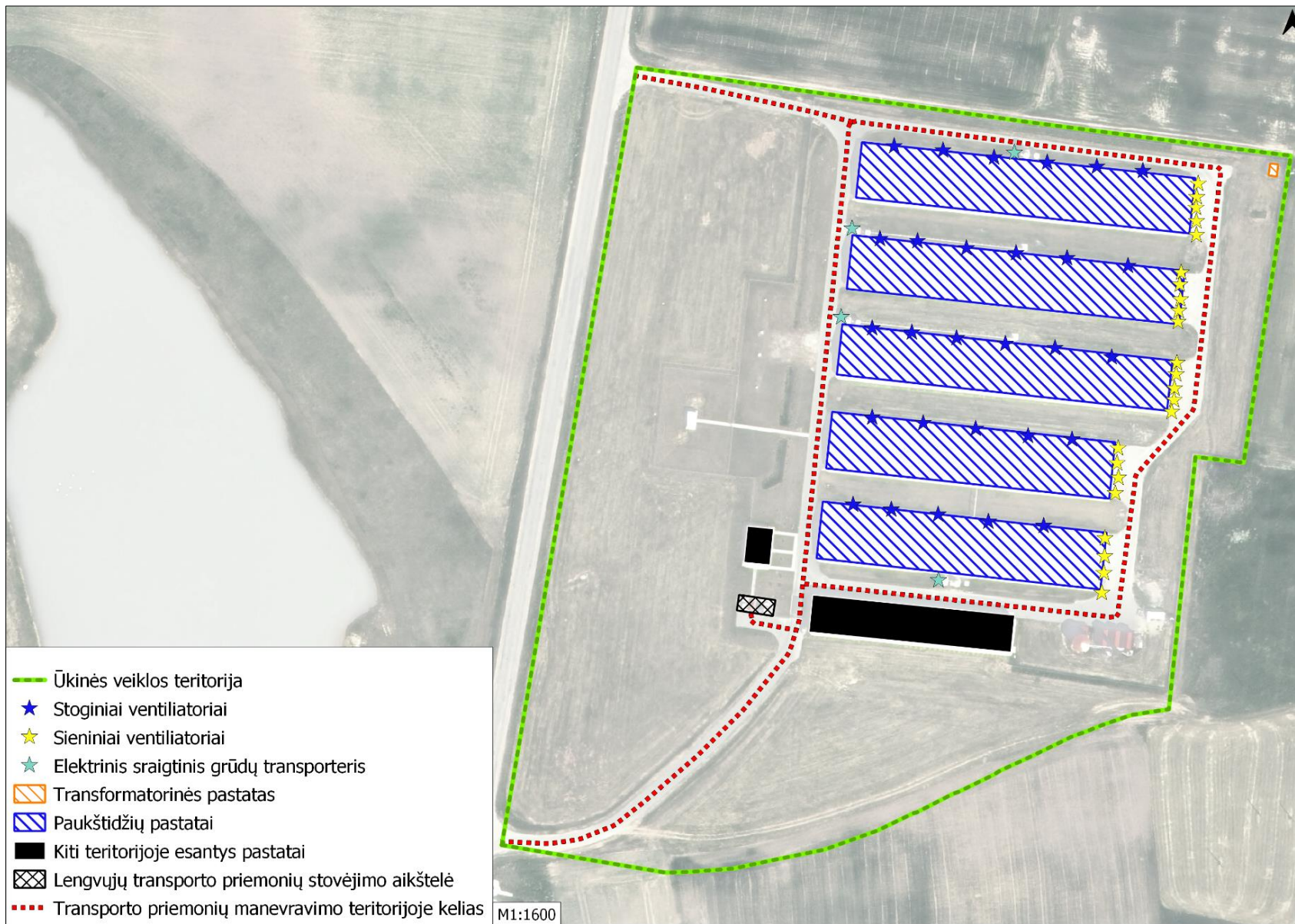
5 pav. Triukšmo šaltinių išsidėstymas ūkinės veiklos teritorijoje
